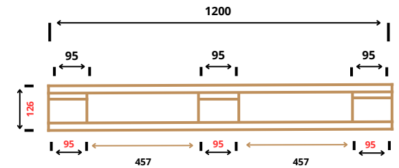
DIMENSIONES GENERALES EN MILIMETROS - VISTA FRONTAL
