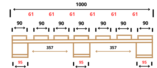
DIMENSIONES GENERALES EN MILIMETROS - VISTA LATERAL
