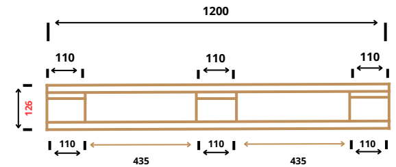
DIMENSIONES GENERALES EN MILIMETROS - VISTA FRONTAL
