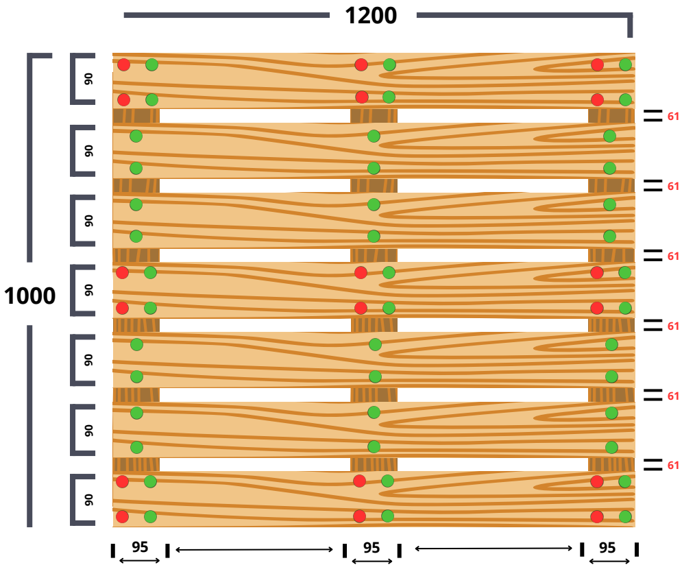
Dimensiones generales en milímetros - Vista de Planta
